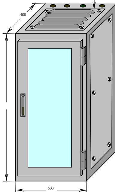
Шафа з обладнанням ІКМ4х30, модемами WATSON5, гарантованим живленням, кросом.
