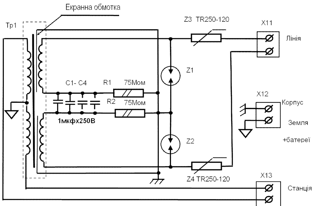
Рис.1 Електрична схема пристрою ЛУП 600/600ПЛЗ
