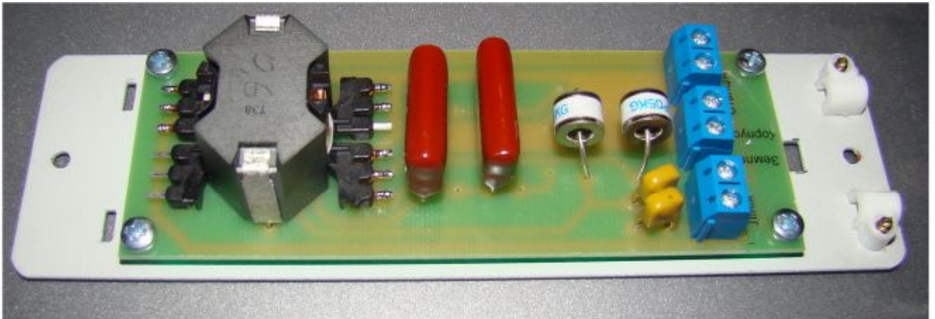
ЛУП 600/600 ПЛЗ без кожуха
